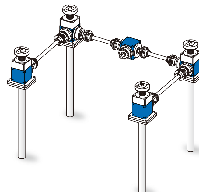
四軸U型升降機 (選配頂板、護管)
