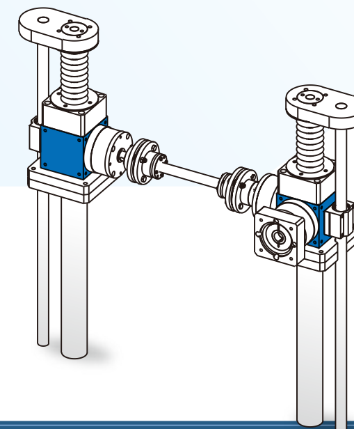
雙軸升降機 (選配頂板、線性導桿、護管)
