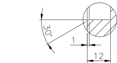
a 細部放大圖 2:1
